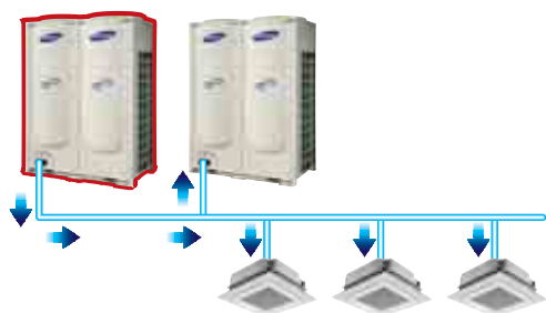
Заправка хладагента
